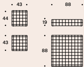
Tavolini / Low tables
