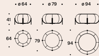
Poufs con telaio / Poufs with frame
