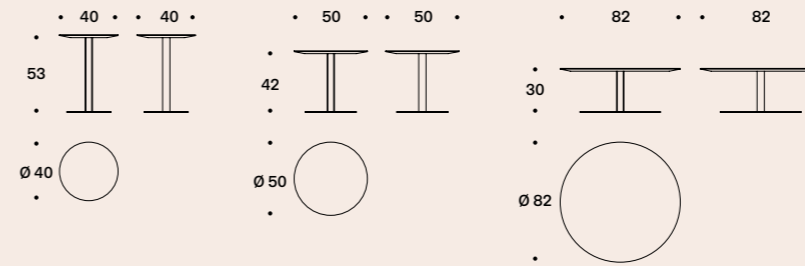
Tavolini / Low tables
