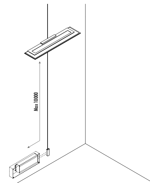
KIT DI ALIMENTAZIONE REMOTO / REMOTE POWER SUPPLY KIT
